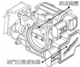
節流閥體
