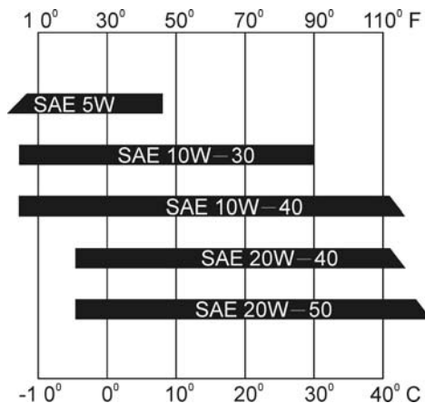
機油適用溫度表
