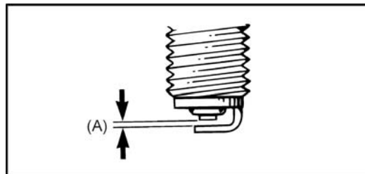
(A) 火星塞間隙
