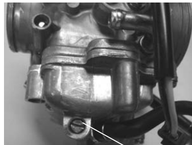
洩油螺絲
