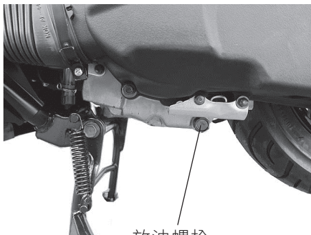
放油螺栓
