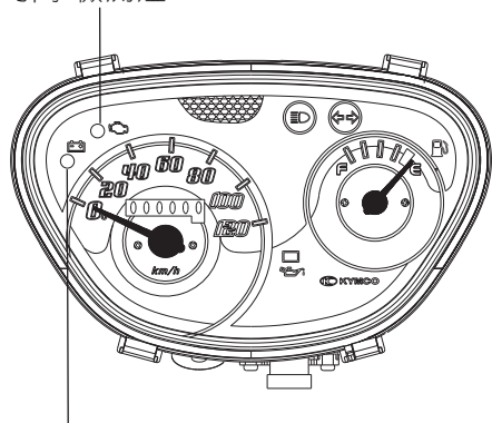
電瓶低電壓警示燈
